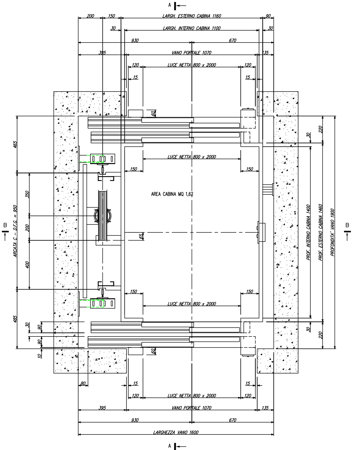
PIANTA VANO SCALA 1:10
